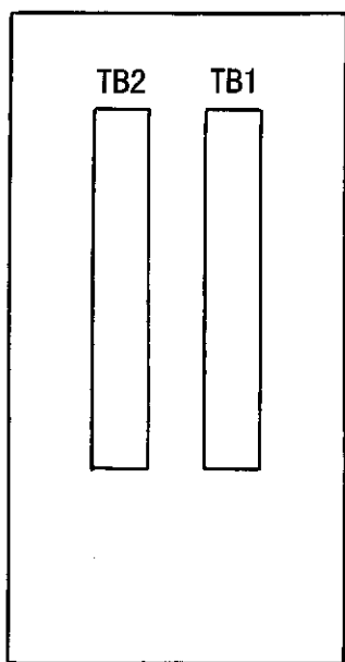
AN-3196 背面端子图
